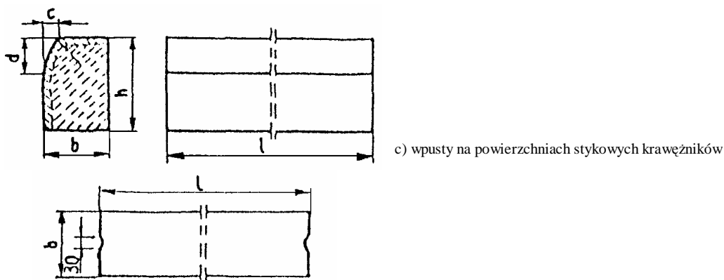
Rys. 1. Wymiarowanie krawężników
